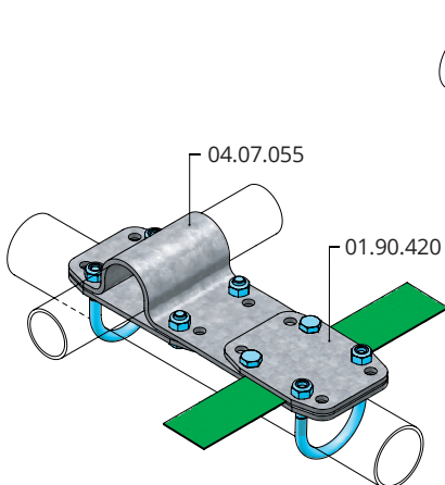
Keerband op schoftboombeugelklem
