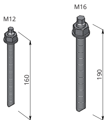
Ankerstang, standaard
