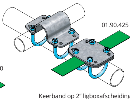
Keerband op 2" ligboxafscheiding
