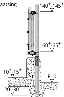
Doorsnede plaatsing
