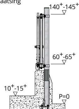
Doorsnede plaatsing
